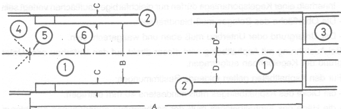
Abbildung 13: Kugellaufbereich - Ausführung mit Fehlwurfrinnen
