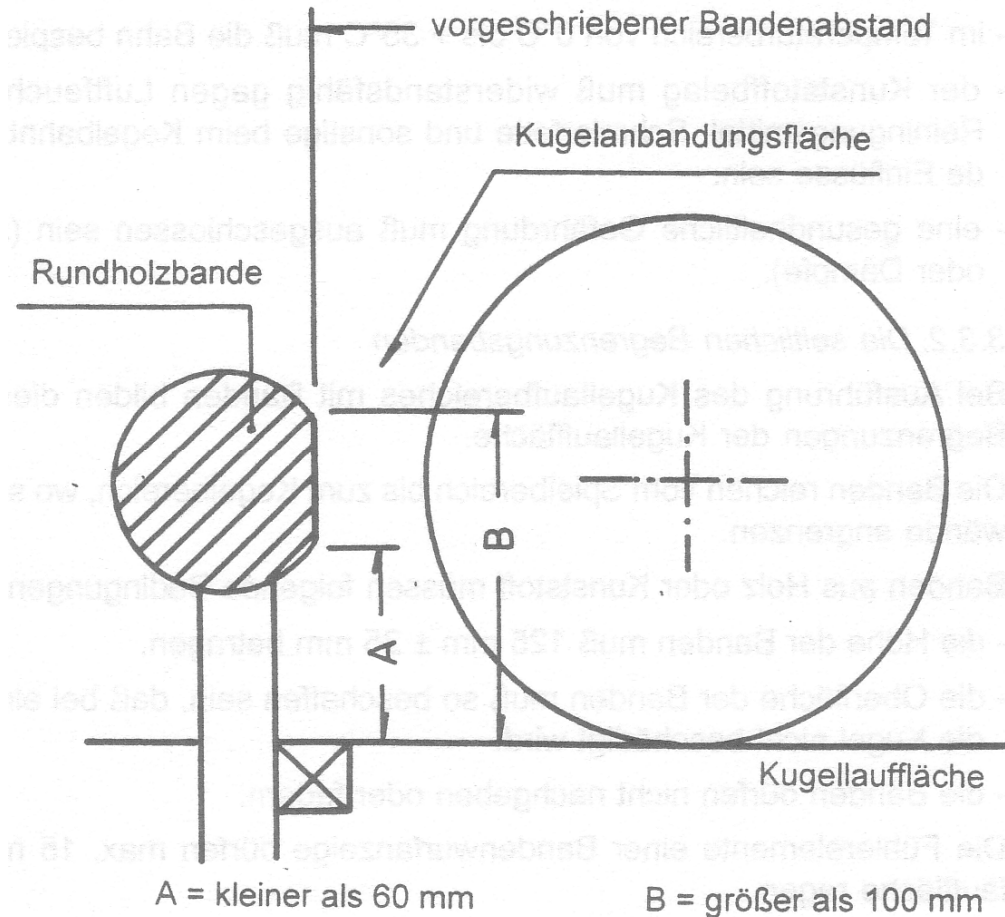
Abbildung 18: Ausführungen der Rundholzbanden
