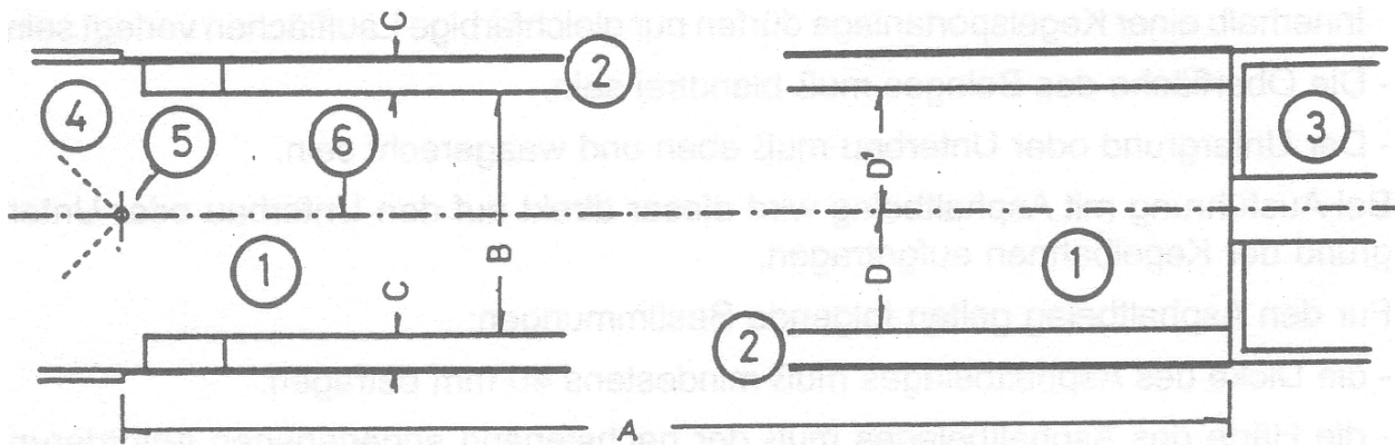
Abbildung 14: Kugelaufbereich - Ausführung in Segmentbauweise
