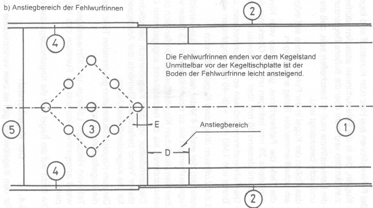
Abbildung 19: Ausführungsmöglichkeiten für Fehlwurfrinnen
