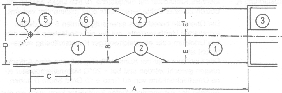
Abbildung 12: Kugellaufbereich - Ausführung mit Banden
