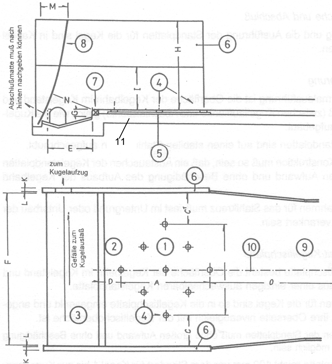
Abbildung 20: Die Kegelstandfläche in Normalausführung
