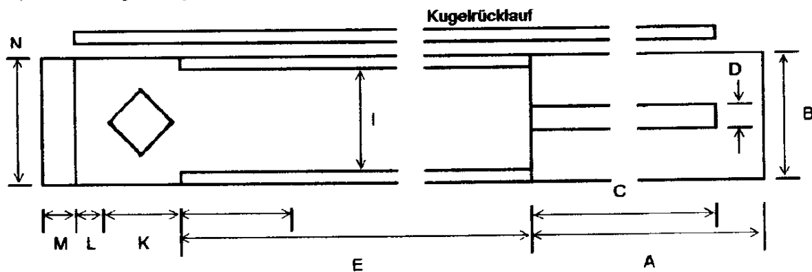
Abbildung 10 Hauptabmessungen einer Bahneinheit
