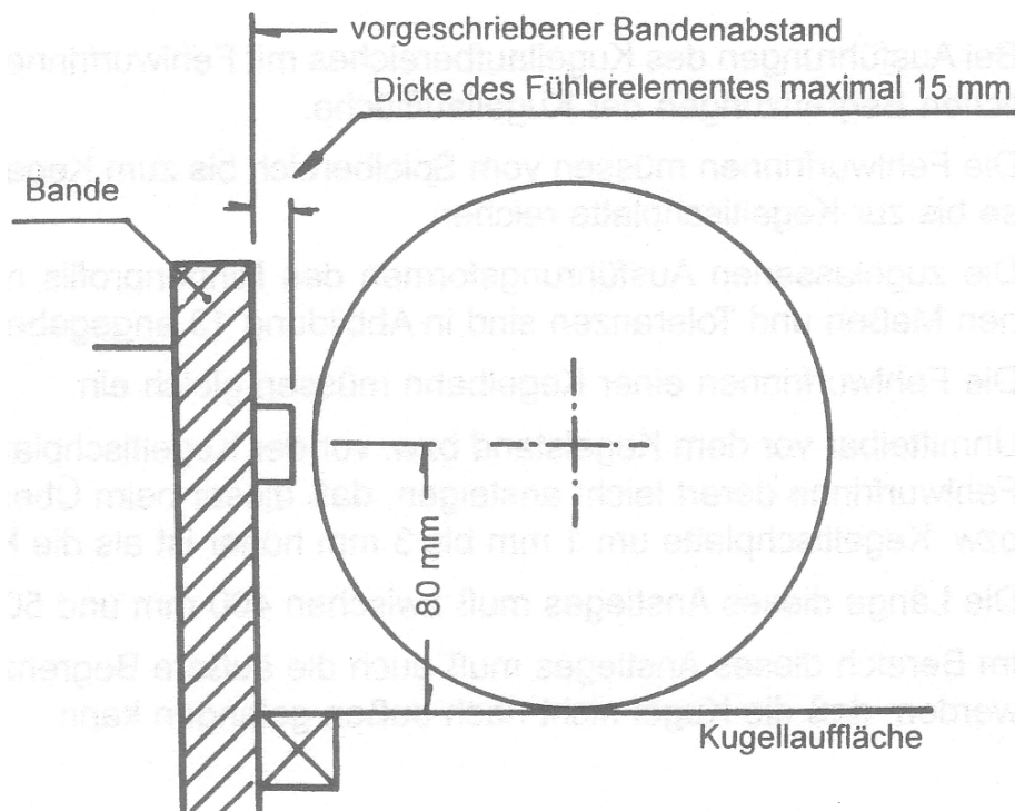
Abbildung 17: Anordnung der Fühlerelemente der Bandenwurfanzeige
