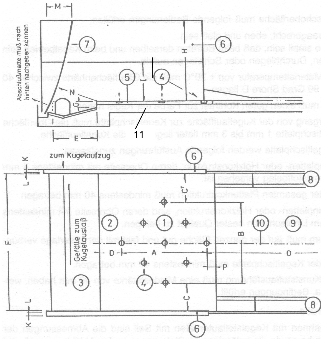
Abbildung 21: Der Kegelbereich bei Ausführung mit Kegeltischplatte und Fehlwurfrinnen
